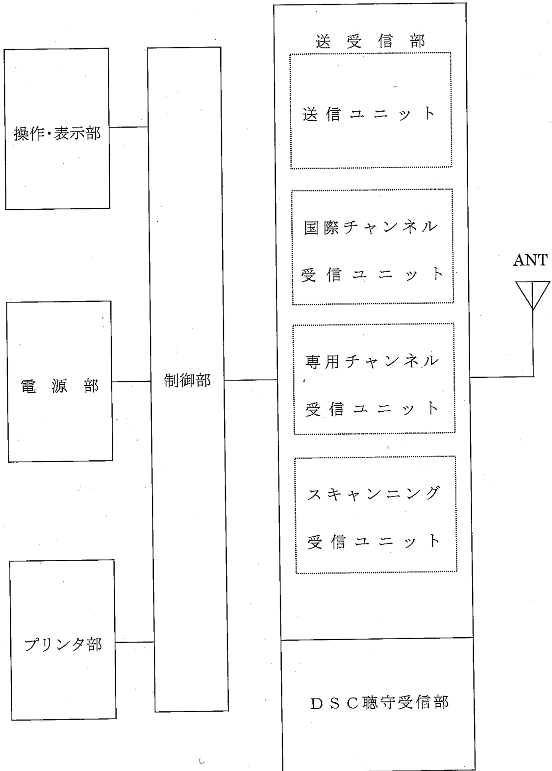
別図 MS-CVS10C/FMブロックダイヤグラム
