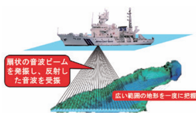
測量船による海底地形調査
