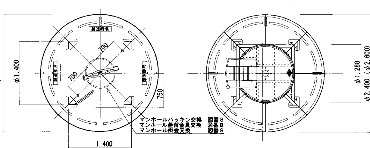
浮体平面図 (A-A')
