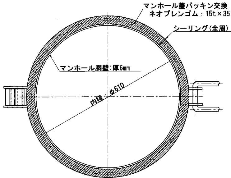
マンホールパッキン詳細図 S=1/10
