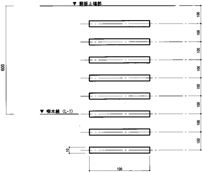
喫水線（目盛）詳細
