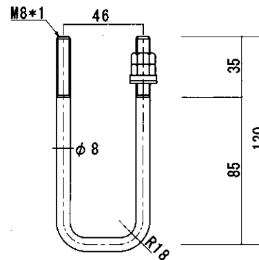
マンホール掛金詳細図 S=1/3
