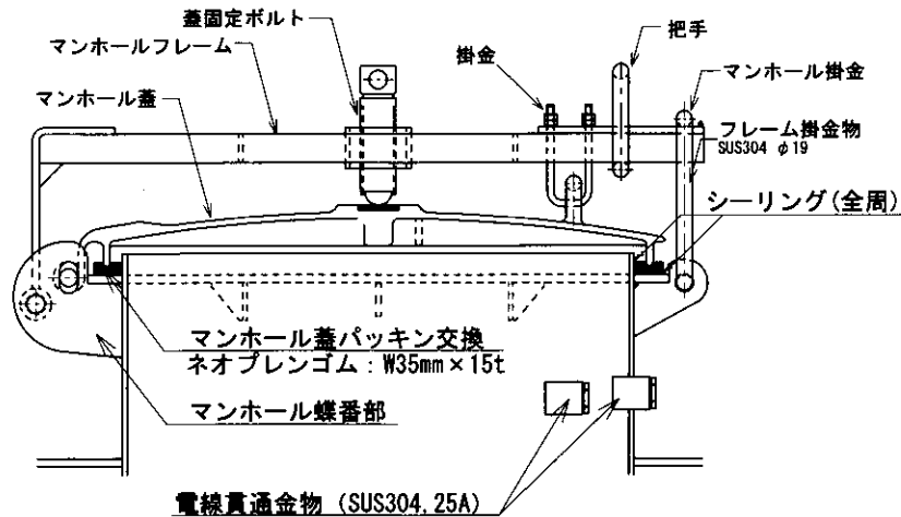
マンホール詳細図 S=1/10
