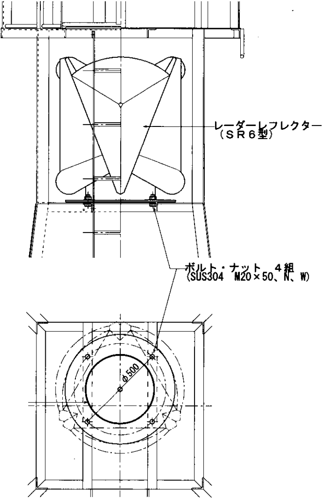
レーダーレフレクター取付詳細図 S=1/20
