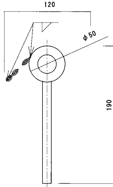
マンホール蓋留金具詳細図 S=1/3
