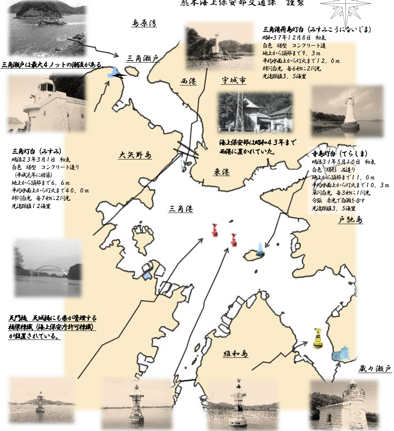
三角港白瀬西灯浮標 (みすみこうしらせにし) 昭和36年12月12日 初点 赤色円すいすい浮標1個付 赤色 やぐら形 水面から灯火まで4.5m モールス符号赤光 毎8秒にA (・―) 光達距離4.0海里
