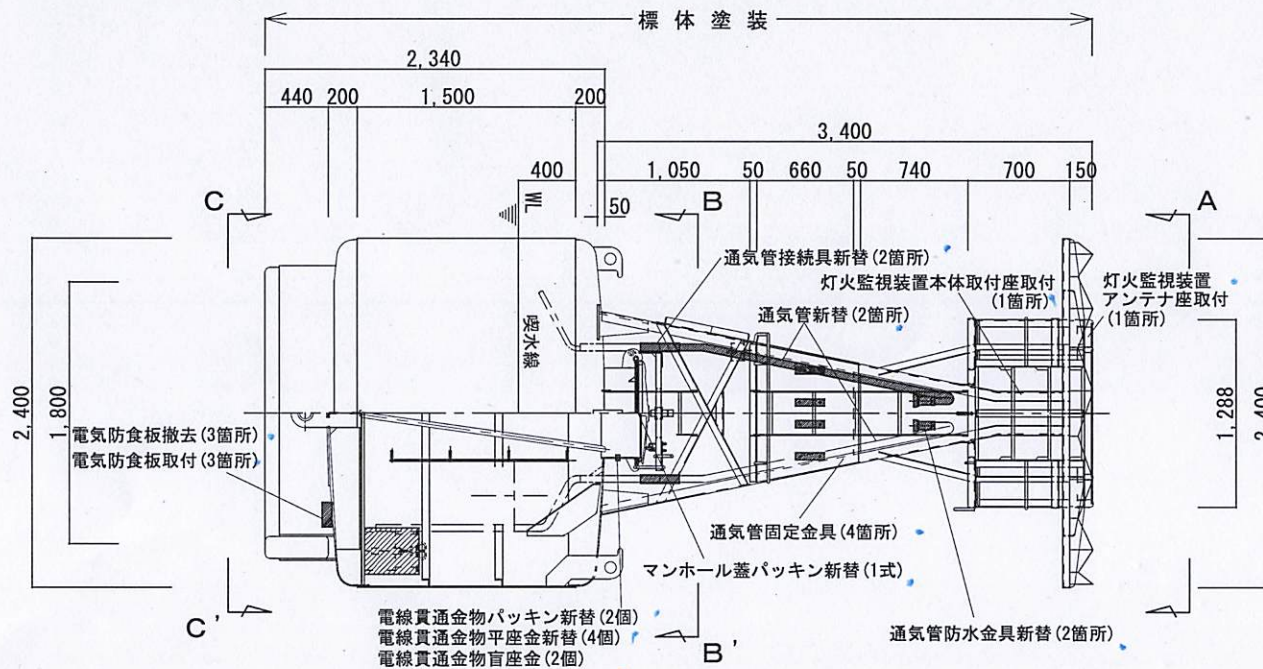
L-U型標体立・断面図
