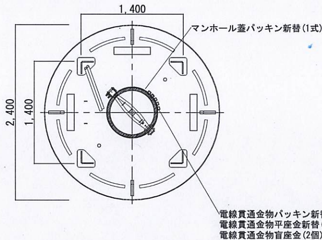
浮体平面図 (B-B')
