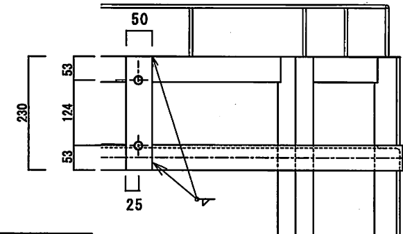
B 詳細図
