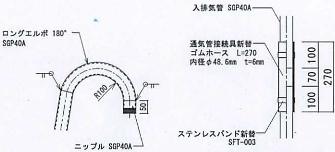
A部詳細図 S=1/10
