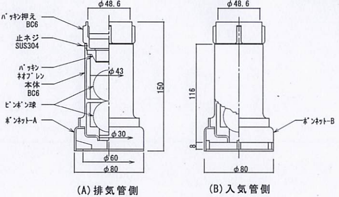
通気管防水金具詳細図 S=1/3
