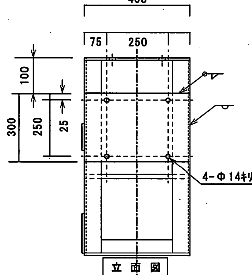
82043 標詳細図 S=1/7
