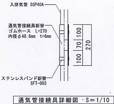
通気管接続具詳細図 S=1/10
