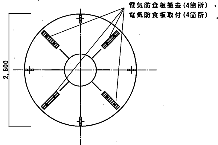
浮体平面図(C-C') S=1/50
