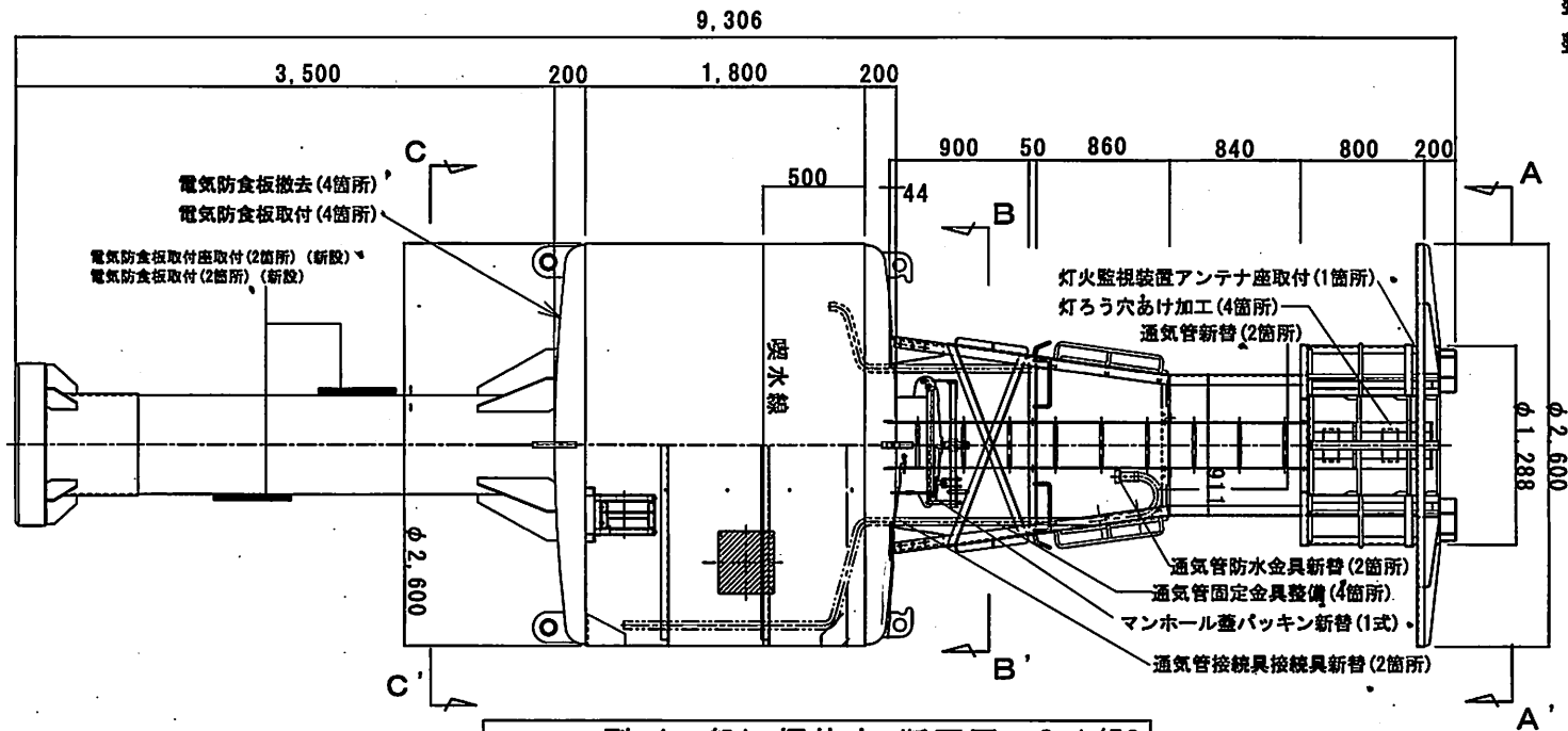
L-1型(一般)標体立・断面図 S=1/50
