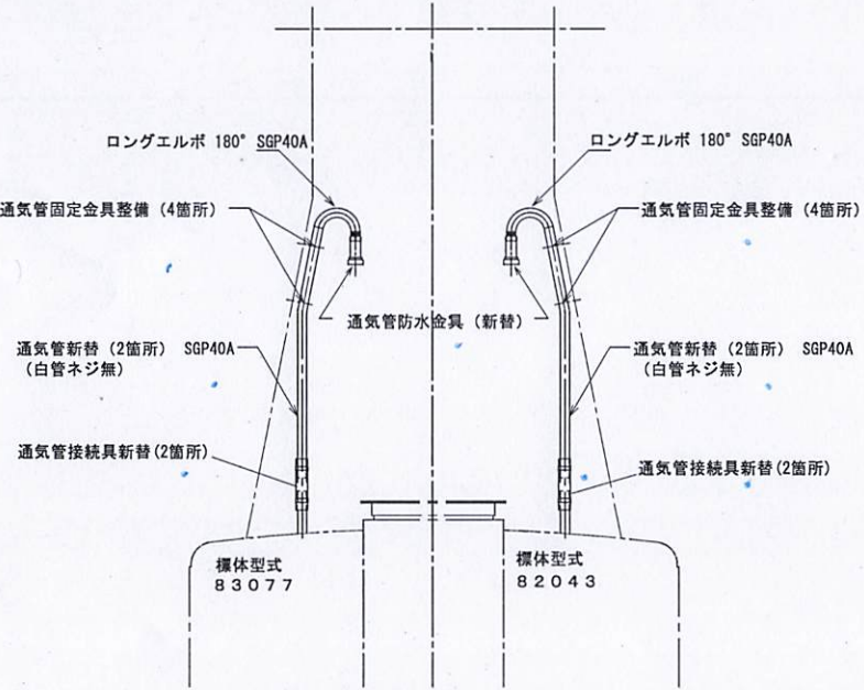
通気管詳細図 S=1/30
