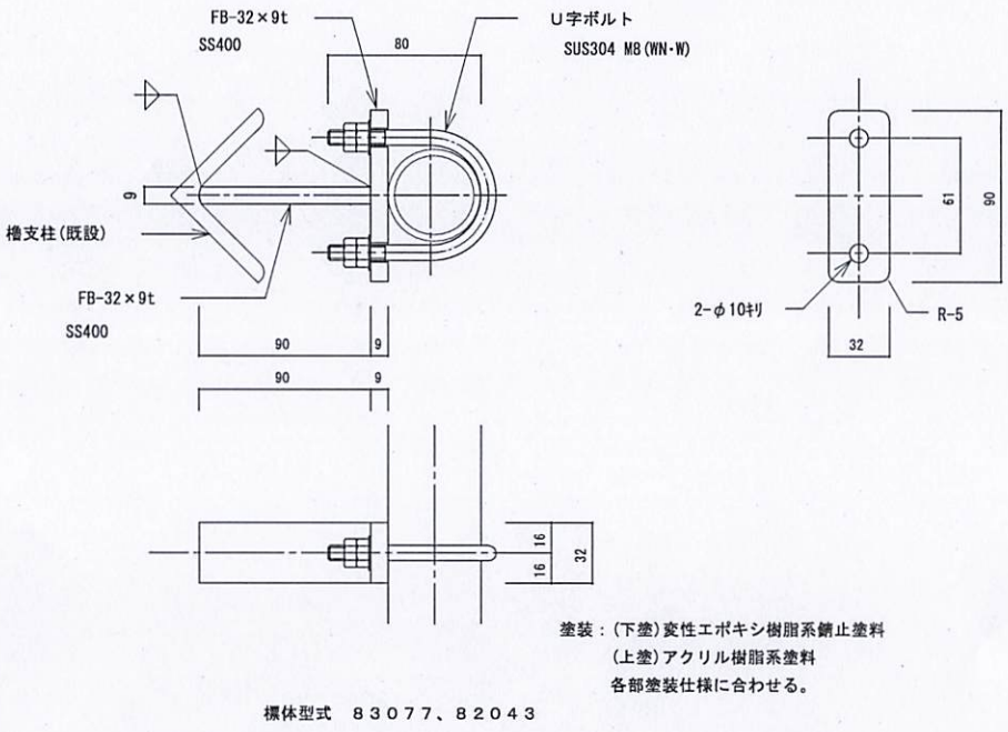
通気管固定金具 S=1/3
