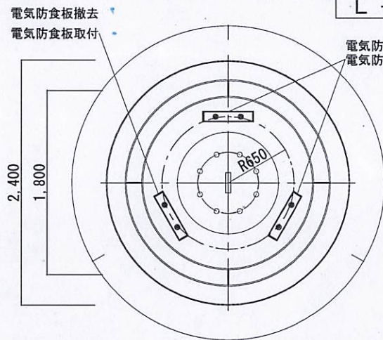
浮体平面図 (C-C')
