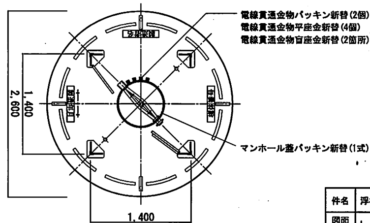
浮体平面図(B-B') S=1/50
