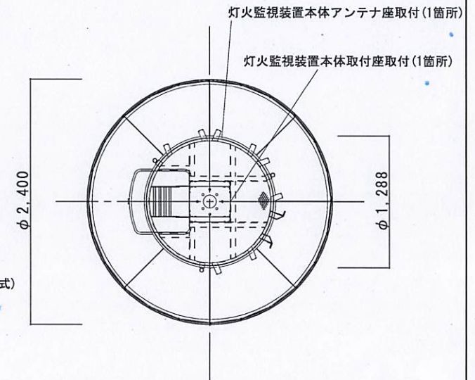
檣平面図 (A-A')
