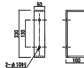
83077アンテナ取付座詳細図 S=1/10
