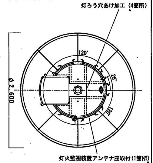
標体平面図(A-A') S=1/50
