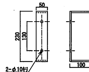
82043アンテナ取付座詳細図 S=1/10
