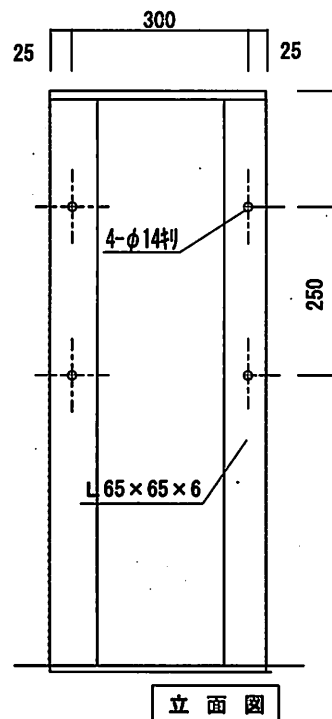
83077 標詳細図 S=1/10
