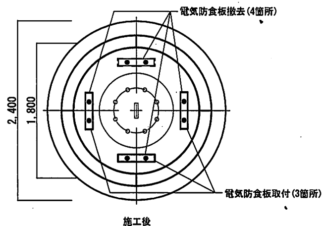
浮体平面図 (C-C')
