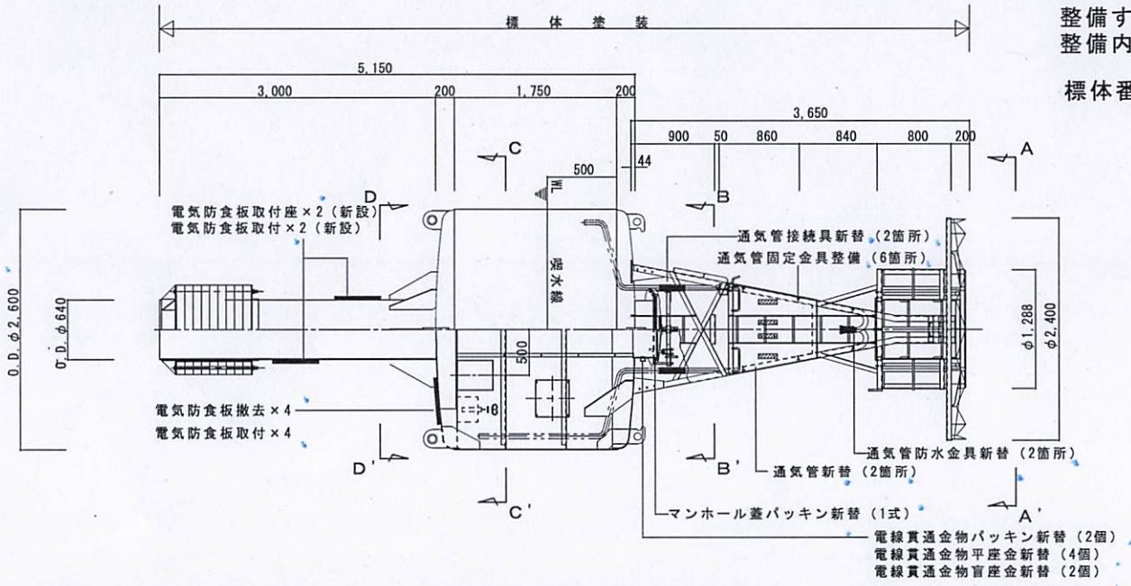
L-1型 (一般) 標体立・断面図
