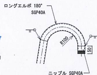
A部詳細図 S=1/10
