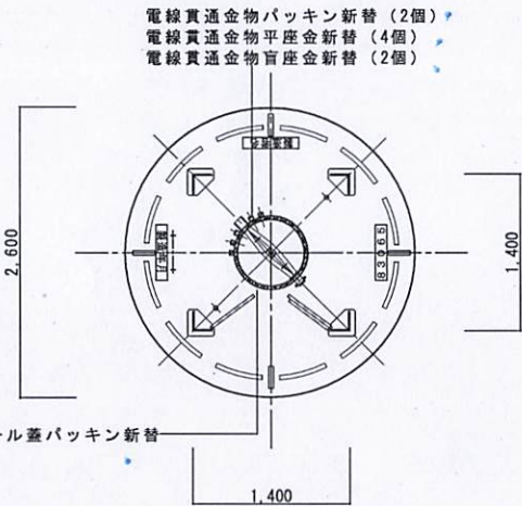
浮体平面図 (B-B')
