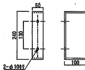
82038アンテナ取付座詳細図 S=1/10
