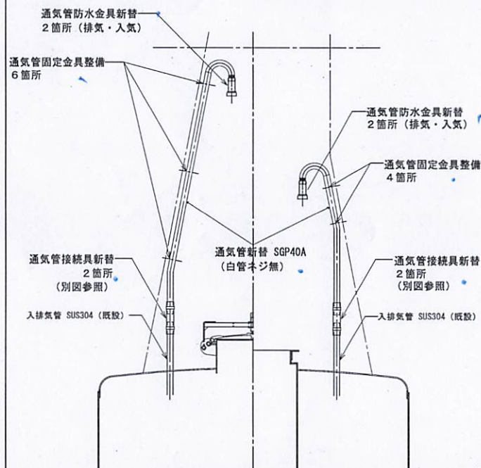
通気管詳細図 S=1/30
