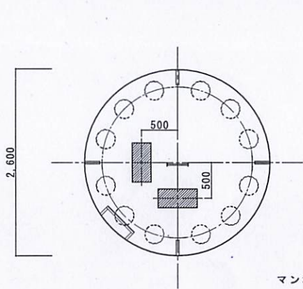
L-1型 (一般) 標体立・断面図
