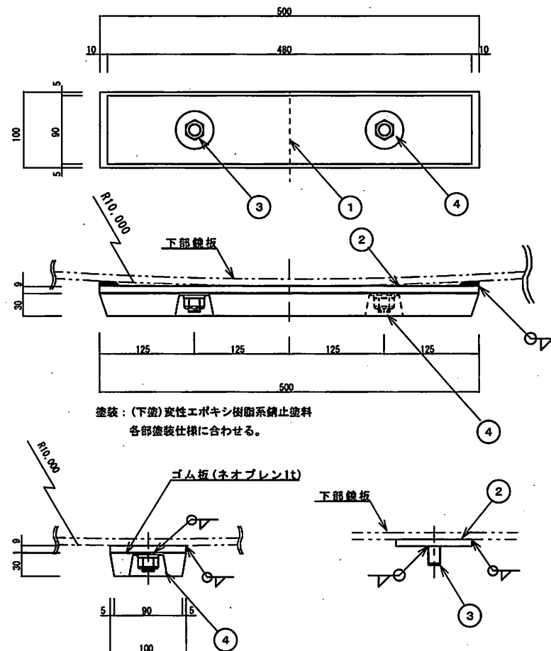
電線防食板取付図 S=1/5
