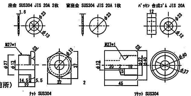
各部品寸法図
