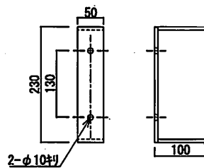
83065アンテナ取付座詳細図 S=1/10
