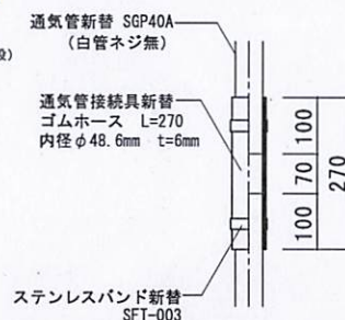
通気管接続具詳細図 S=1/10
