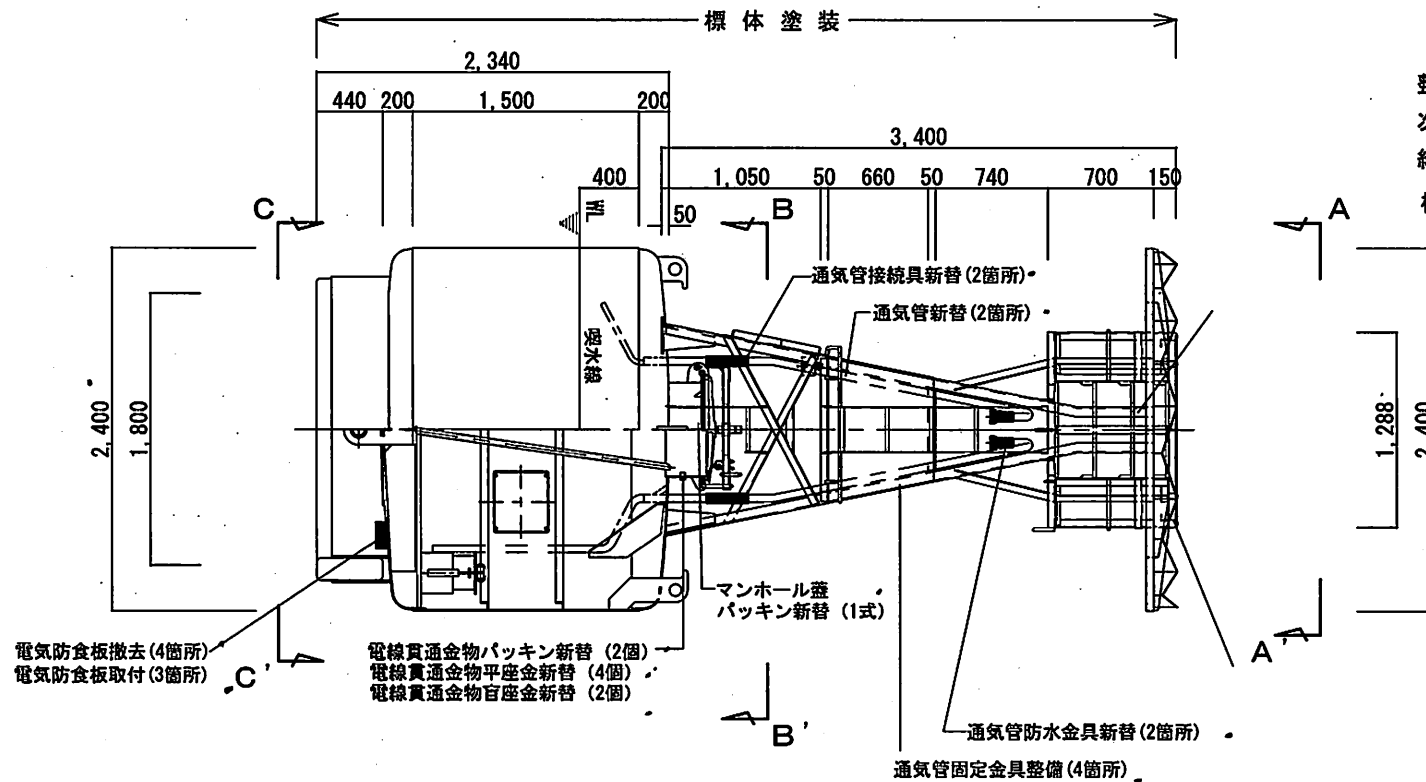
L-U型標体立・断面図
