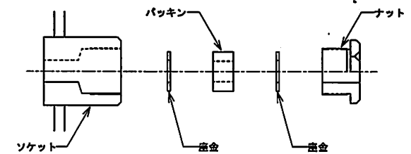
電線貫通金物組立図
