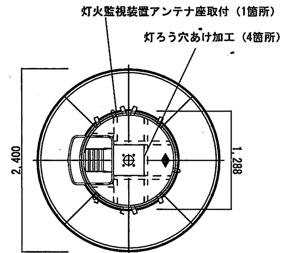
檣平面図 (A-A')
