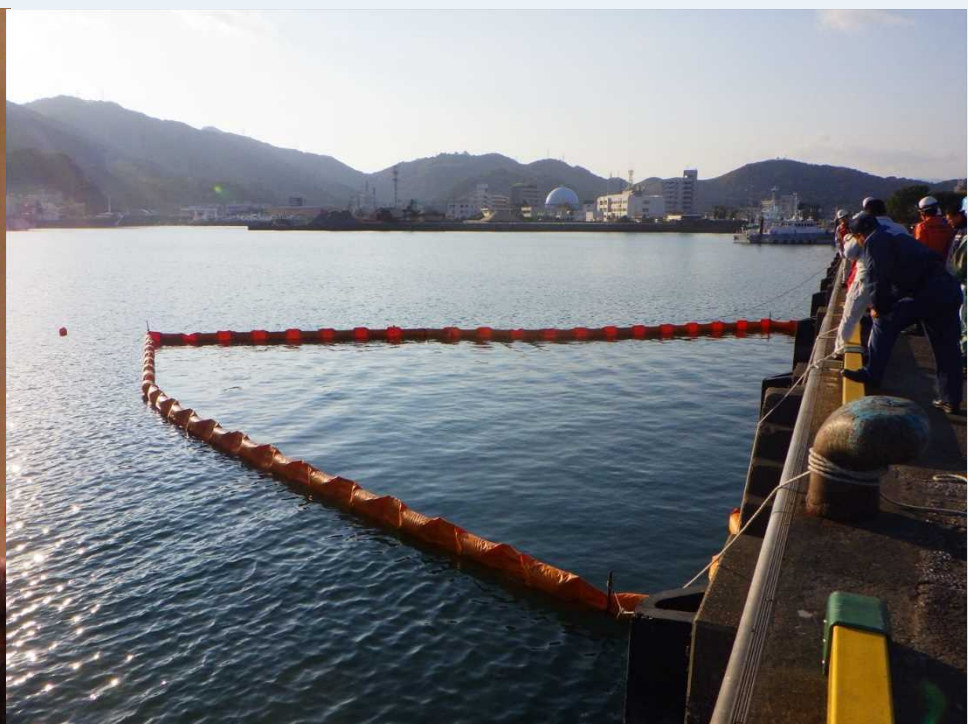
オイルフェンス展張訓練
