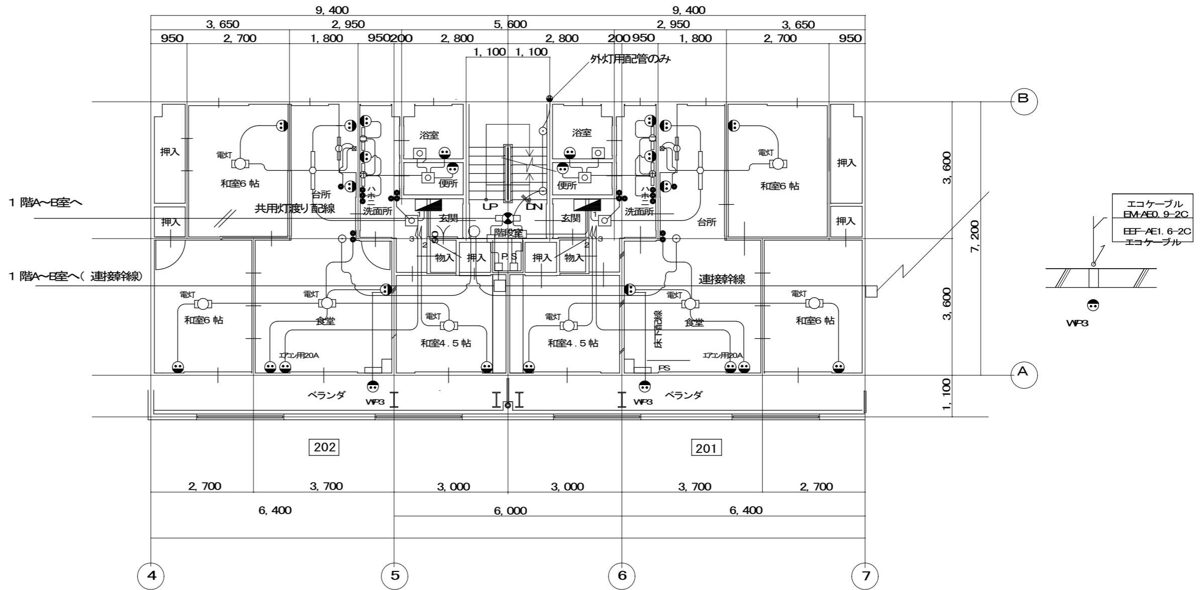
201・202室電気設備配線図 S=1:100
