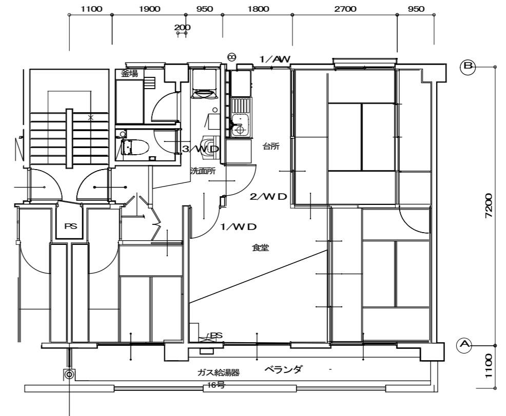
建具キープラン
