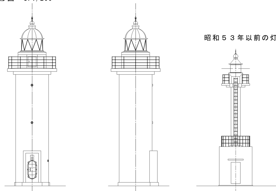
灯塔外形図 S. 1/200
