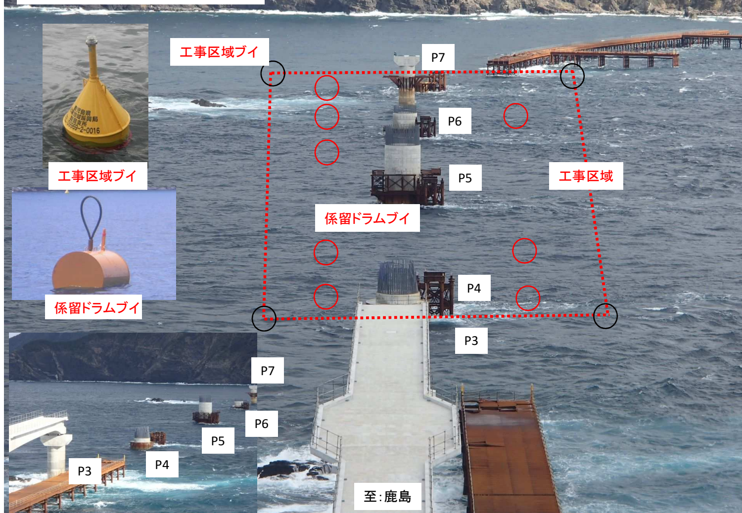
藺牟田瀬戸架橋現場状況(H25年12月)
