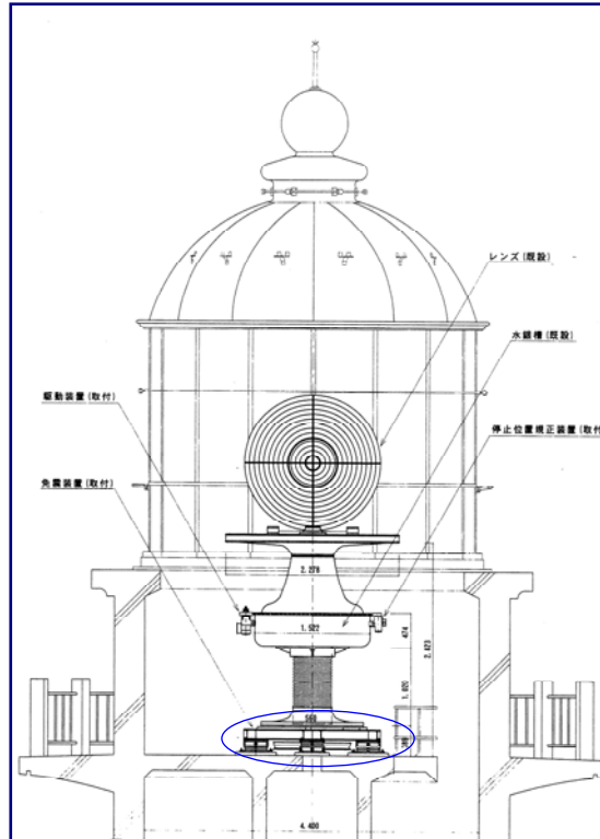
免震装置取付図
