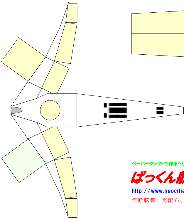
水平スタビライザー
