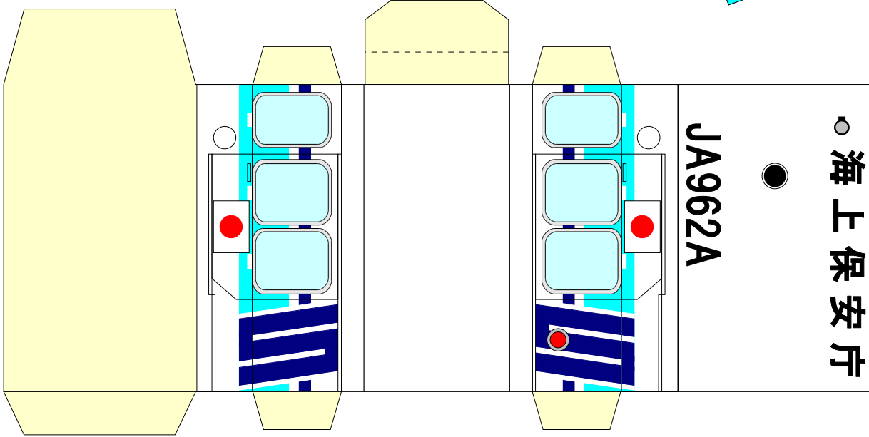
エマージェンシーフロート
