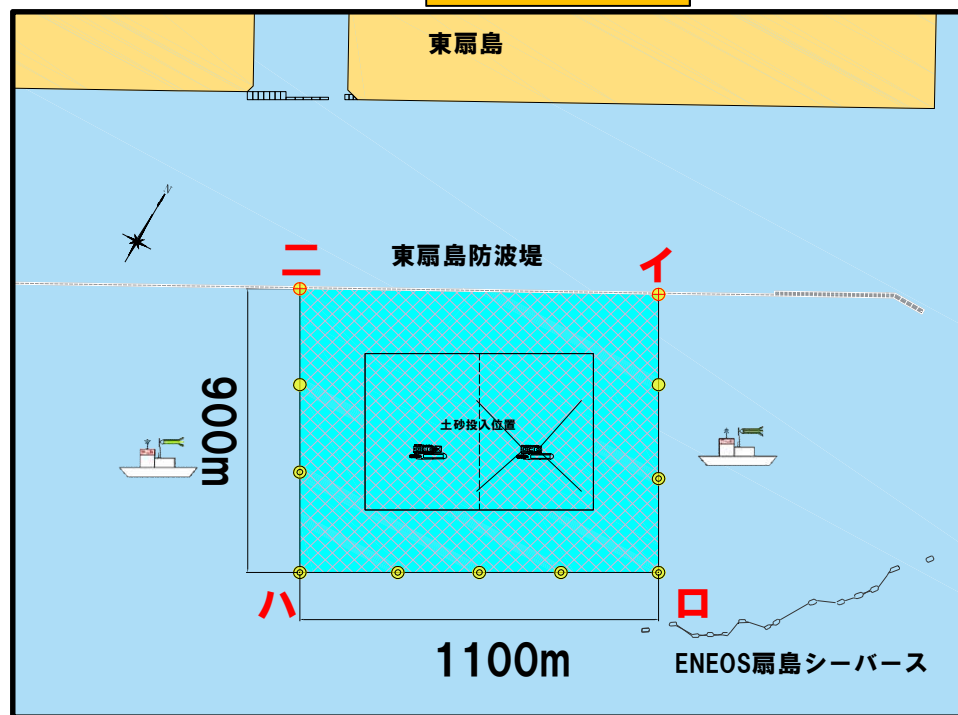
図-2 工事区域図
